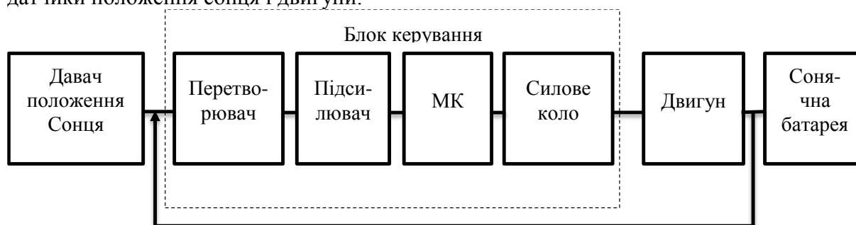
Рисунок 1. Блок-схема управління системи позиціонування
