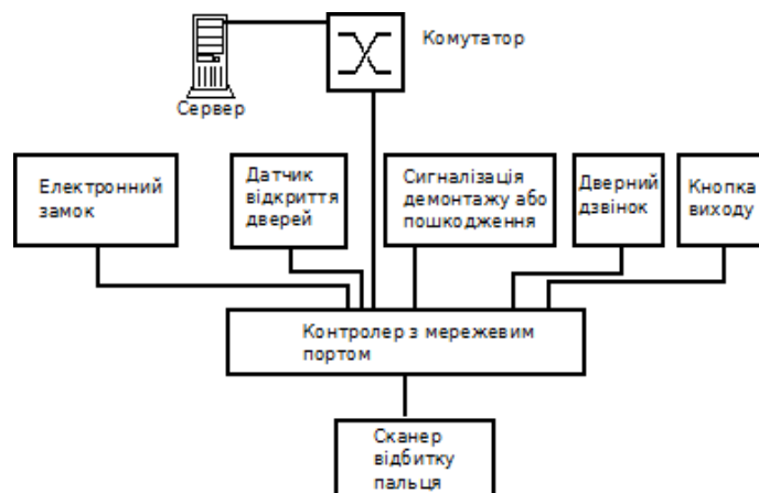
Рисунок 1. Типова схема системи біометричного контролю
