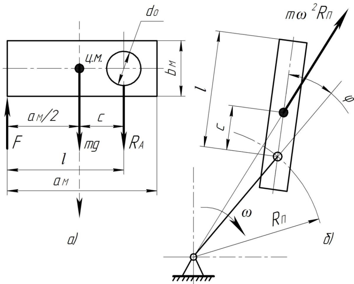
Рисунок 17 – Сили, що діють на молоток дробарки (а) і схема роботи молотка, як фізичного маятника з тертям у шарнірі (б)
