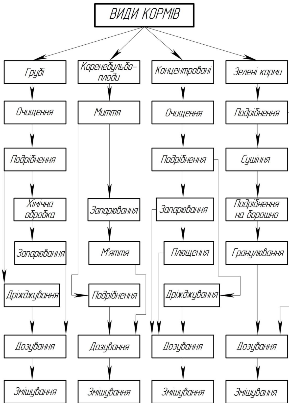
Рисунок 6 – Технологічна схема обробки і приготування кормів
