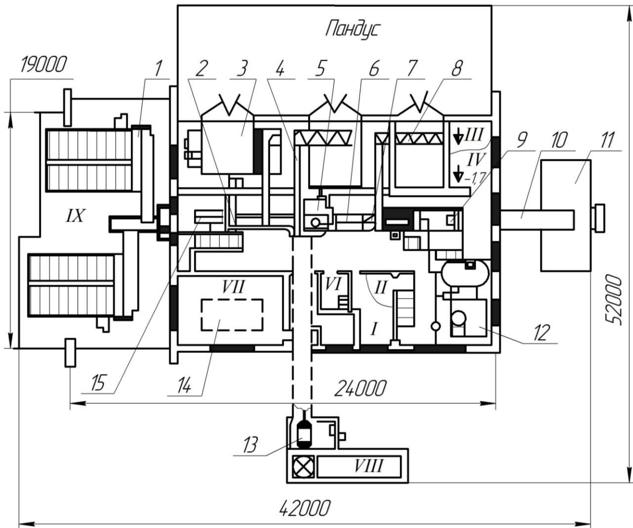
Рисунок 9 – План кормоцеху КЦК-5:
