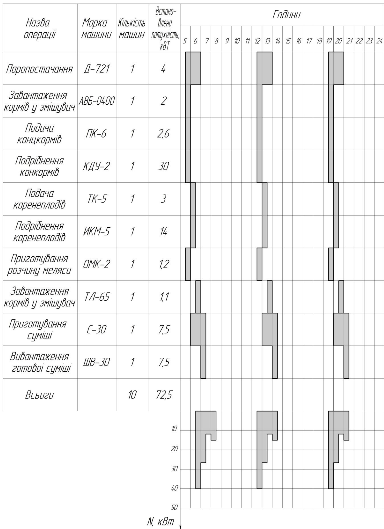
Рисунок 13 – Графік роботи машин кормоцеху і споживання електроенергії
