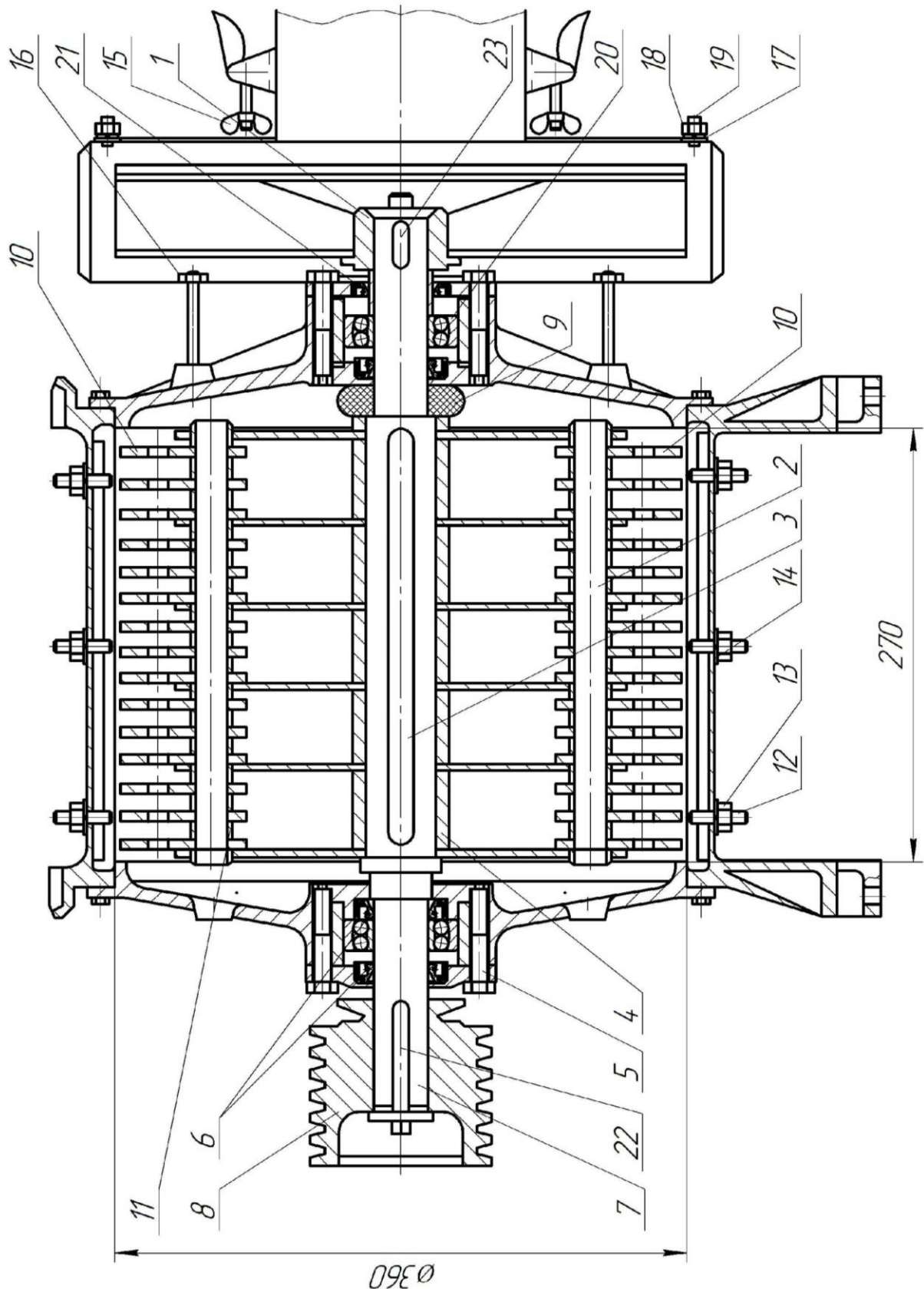
Рисунок 16 – Подрібнювальний апарат кормодробарки:
