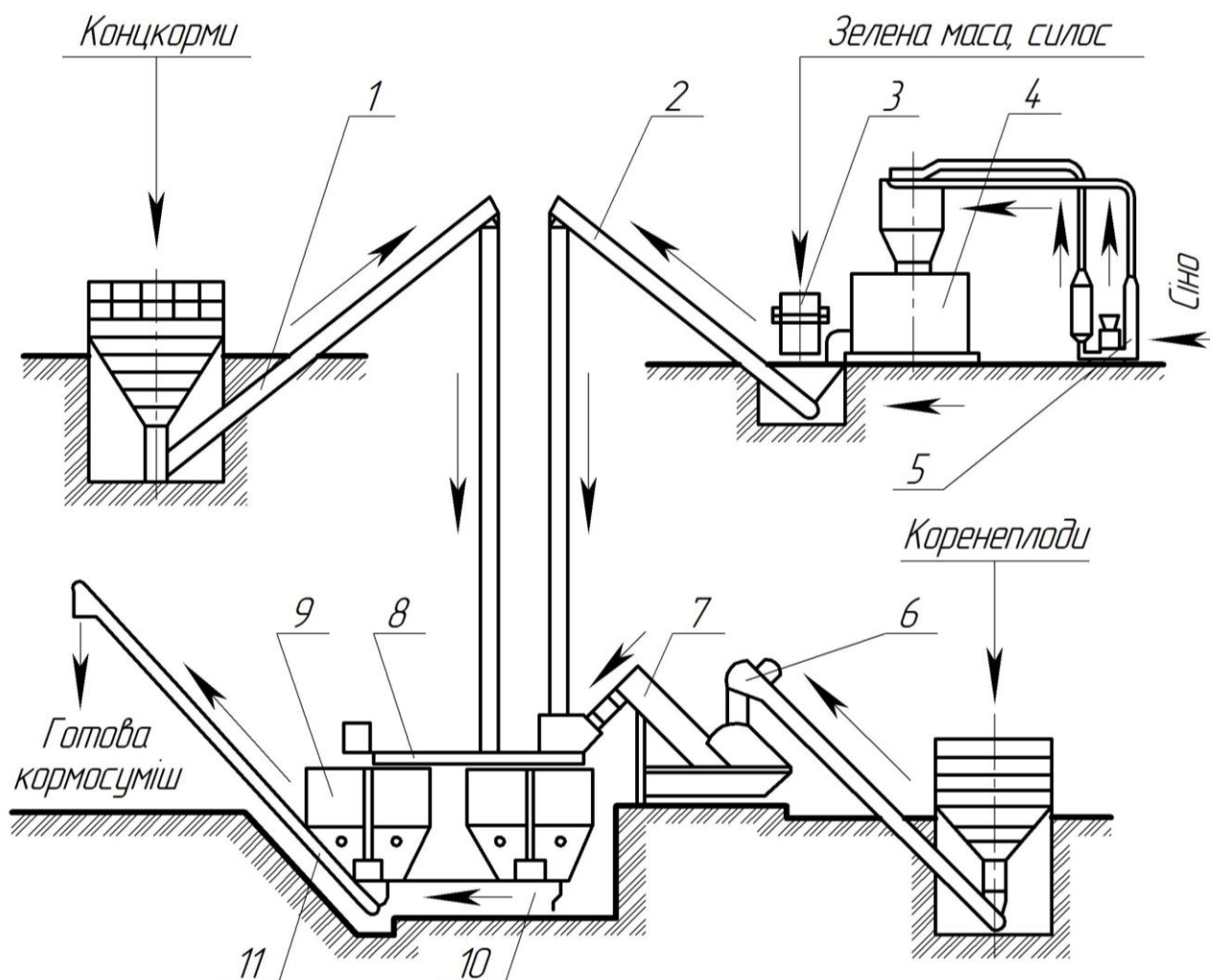
Рисунок 10 – Технологічна схема кормоцеху «Маяк-6» (т.п. 812-116):
