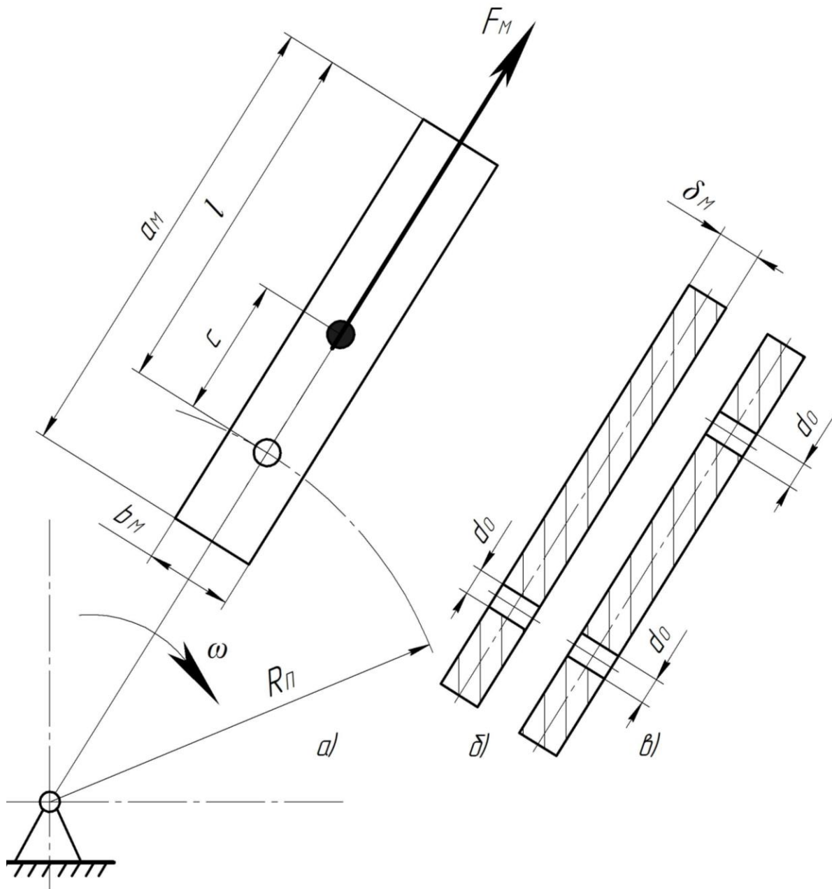
Рисунок 19 – Схема підвісу молотка дробарки та дії на нього відцентрової сили
