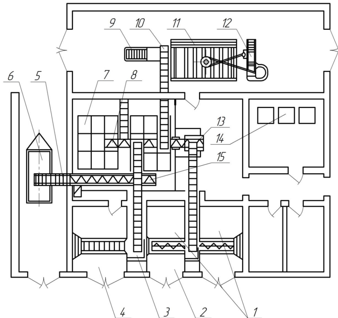
Рисунок 11 – План кормоцеху «Маяк-6» (т.п. 812-116):
