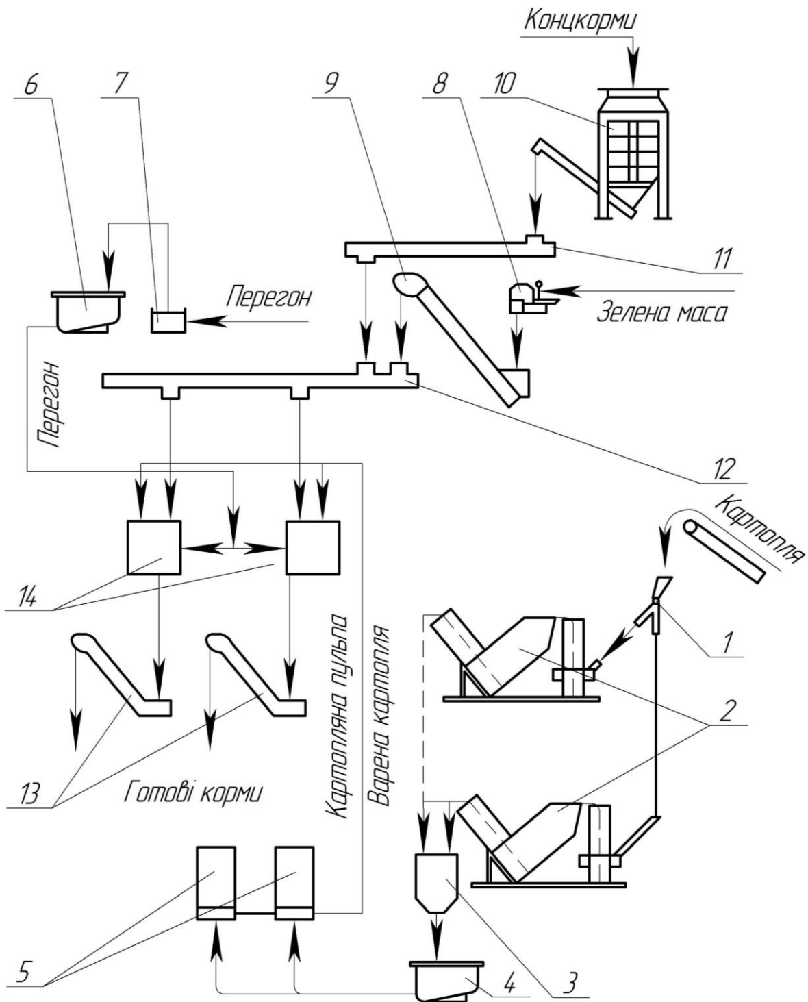
Рисунок 12 – Технологічна схема кормоцеху (т.п. 802-249С):
