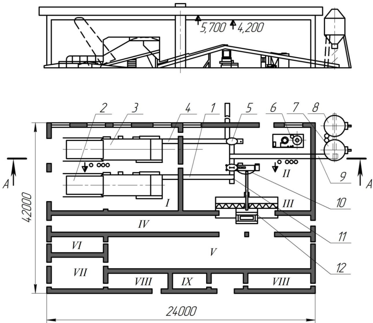
Рисунок 7 – План кормоцеху КОРК-15:
