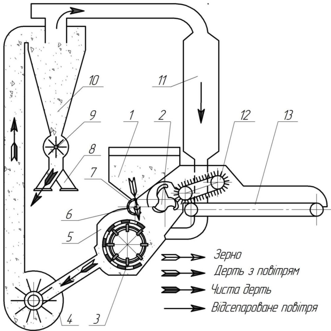
Рисунок 14 – Функціональна схема кормодробарки КДУ-2:
