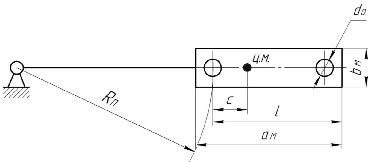
Рисунок 18 – Схема до розрахунку молотків з двома отворами
