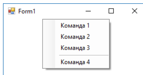
Рис. 10.21. Контекстне меню – об'єкт класу ContextMenuStrip
