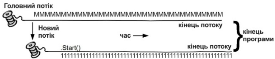
Рис. 12.2. Схематична структура простої двопотокової програми
