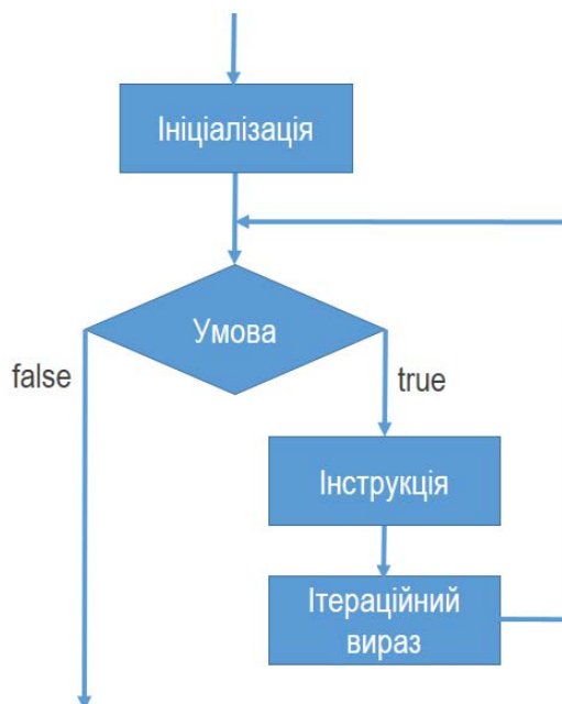
Рис. 2.13. Схеми циклу for
