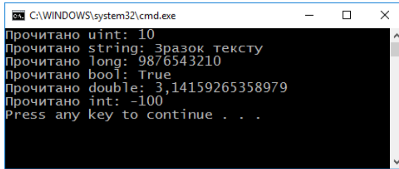
Рис. 11.6. Робота з потоком, що використовує пам'ять як сховище даних
