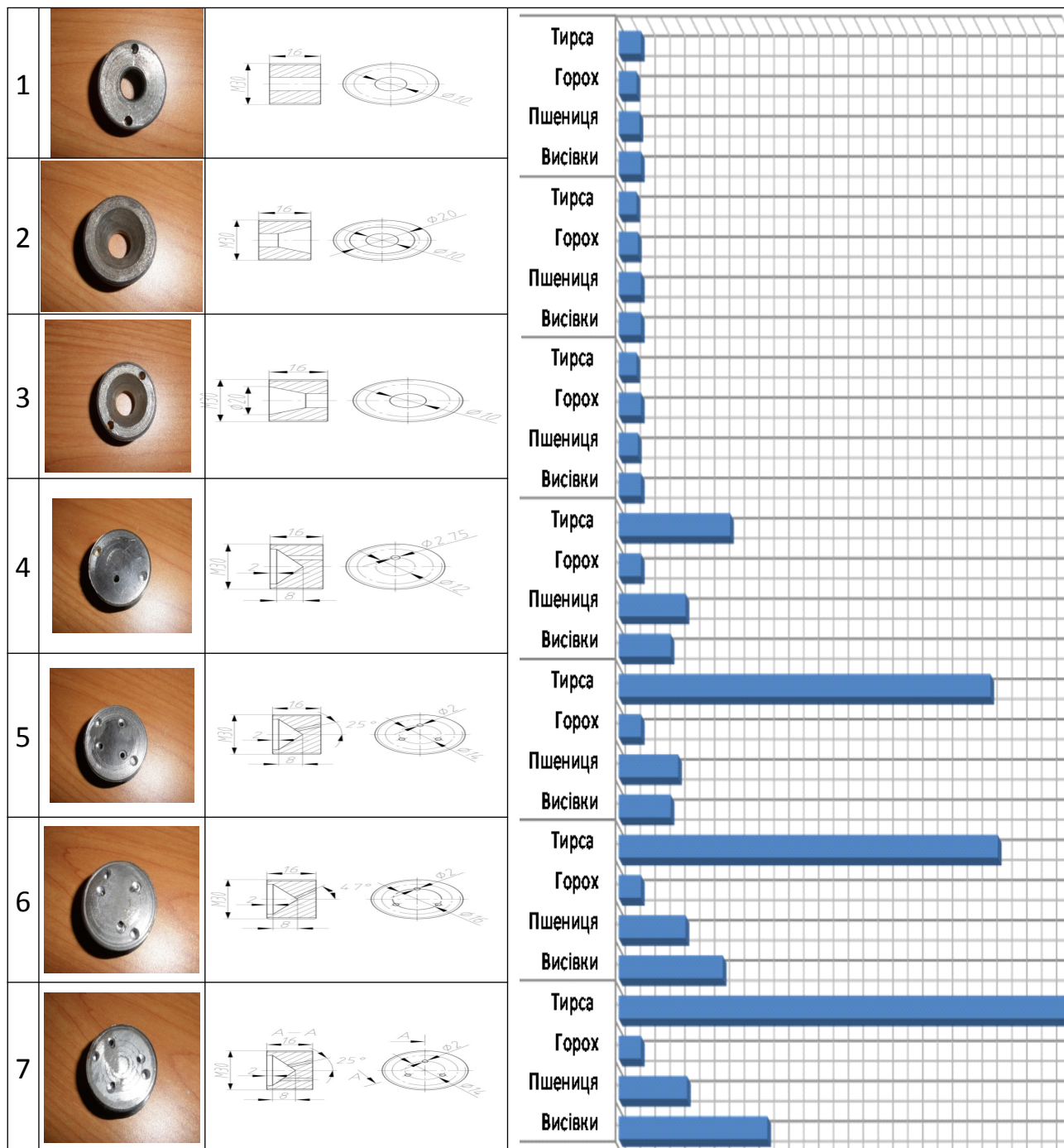
Рис.2. Змінні сопла шнекового пневмомеханічного транспортера: 1, 2, 3 – з центральним отвором різної конусності (діаметр D_{цос} = 10 мм); 4, – з нецентральним отвором (діаметр D_{цос} = 2,75 мм); 5, 6, 7 – з трьома отворами розміщеними з різними кутами до осі
