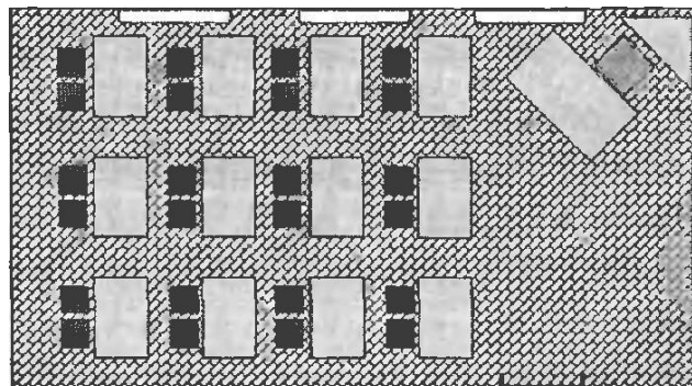
Рис. 2.41. Схема класу
