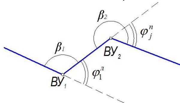
Рисунок 14. Схема визначення кутів повороту траси
