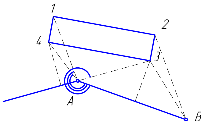
Рисунок 21. Побудова на місцевості проектних осей
