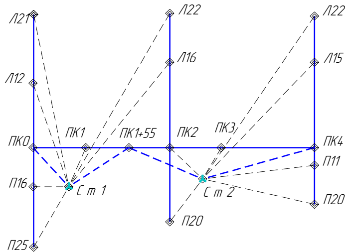
Рисунок 17. Схема нівелювання поперечного профілю
