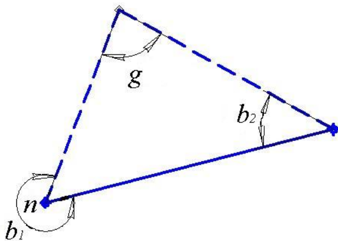
Рисунок 8. Спосіб кутових зарубок
