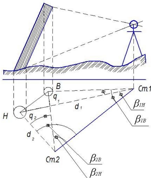
Рисунок 26. Схема визначення нахилу стовпа
