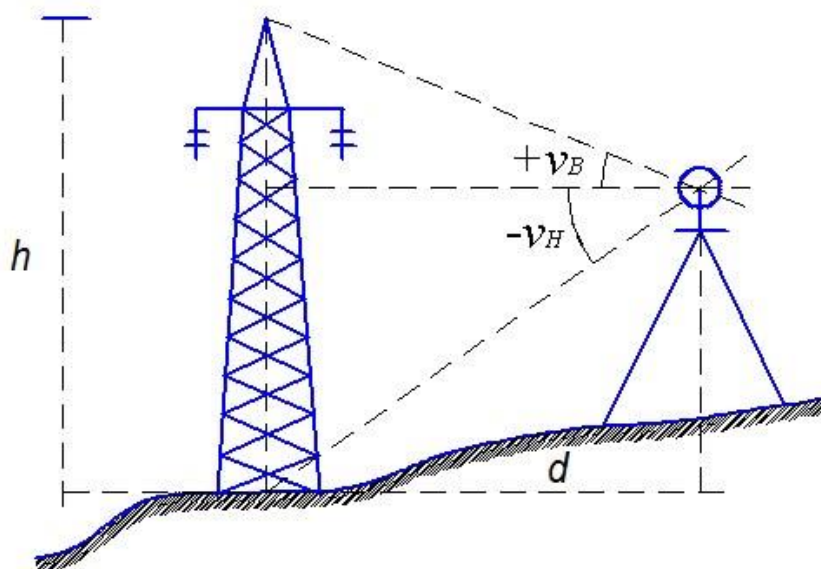
Рисунок 25. Схема визначення висоти споруди
