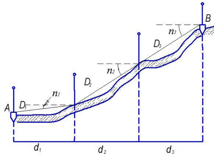
Рисунок 4. Визначення горизонтальних прокладань
