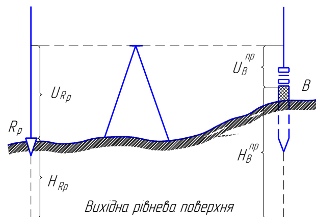
Рисунок 20. Схема побудови проектної оцінки
