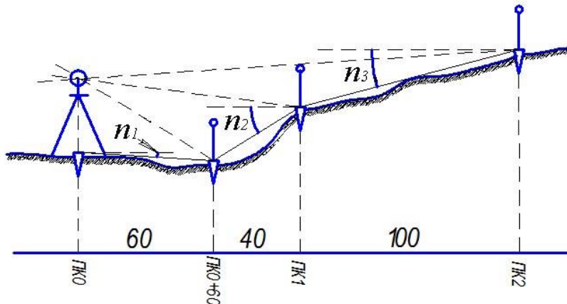
Рисунок 12. Розбивка пікетажу на похилих ділянках траси
