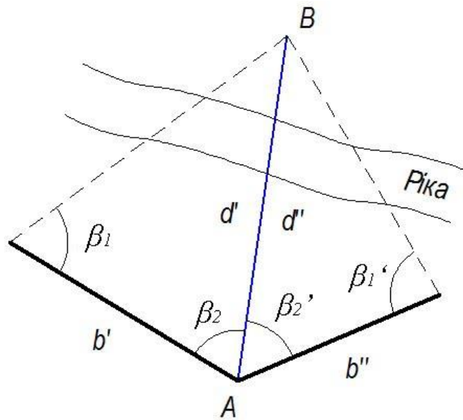
Рисунок 24. Схема визначення недоступної відстані
