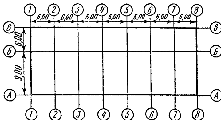
Рисунок 18. План осей споруди
