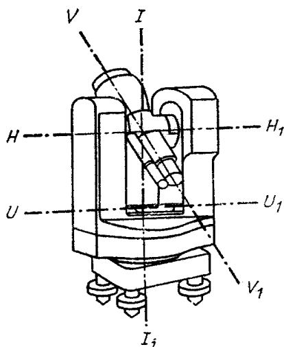
Рисунок 1. Основні осі теодоліта
