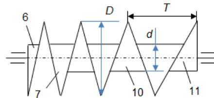
Рис. 2. Схема шнекового
