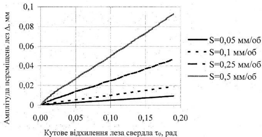
Рис. 2. Графічна залежність амплітуди лезових осциляцій \Delta від несиметричності \tau_\phi положення різальних лез свердла з міжлезовим зв'язком при різних значеннях подачі
