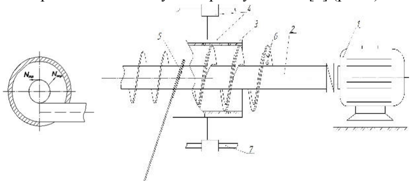
Рис. 3. Спосіб навивання спіралі на крок
