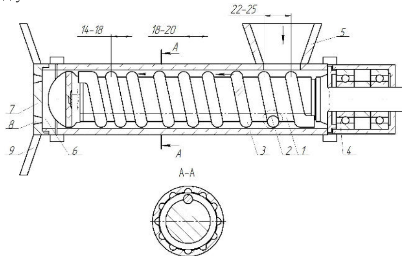
Рис. 1. Гвинтовий робочий орган екструдера
