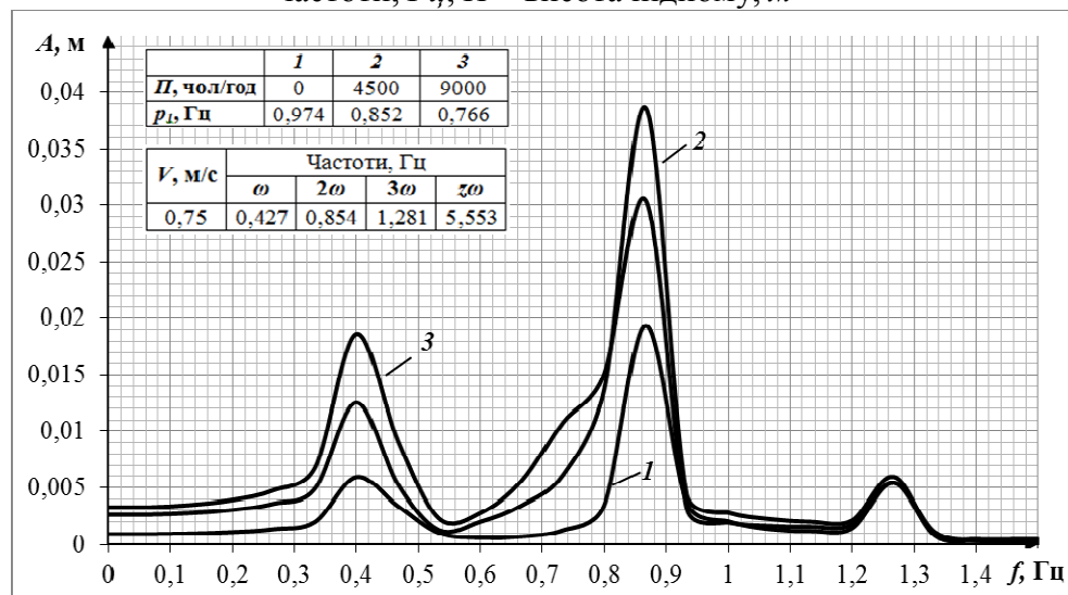
Рис. 2. АЧХ тягового органу ескалатора висотою підйому 45 м при швидкості руху сходового полотна 0,75 м/с
