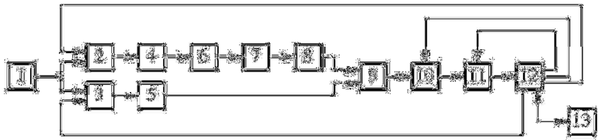
Рис. 1. Система вихрострумової дефектоскопії.
