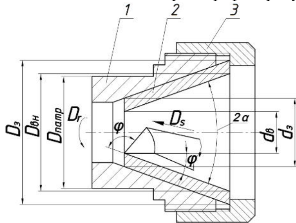
Рис. 1. Схема розточування внутрішньої циліндричної поверхні зразка: 1 – оправка; 2 – дослідний зразок; 3 – накладна гайка
