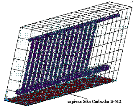
Рис. 2. Тривимірний МСЕ модель симетричної чверті підсиленої вуглепластиковою стрічкою балки
