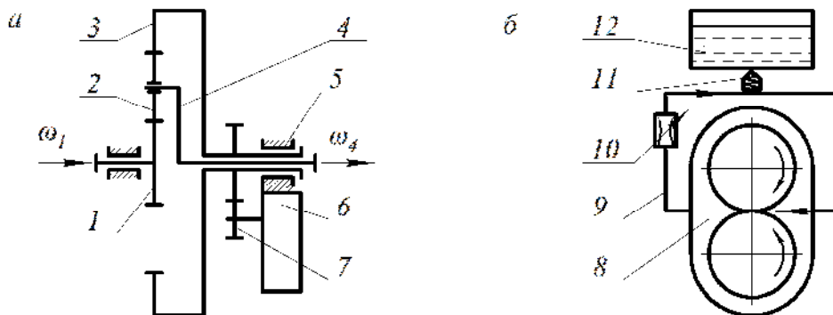
Рис. 1. Схеми: а – зубчастій диференціальної передачі з керуванням через епіцикл та ведучою ланкою – сонячним зубчастим колесом; б – замкнутої гідросистеми
