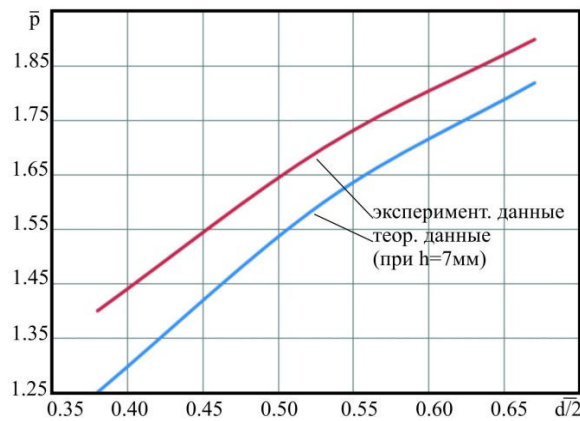
Рис. 3. Порівняльний графік теоретичних і експериментальних даних при комбінованому видавлюванні ( \mu = 0,08 )
