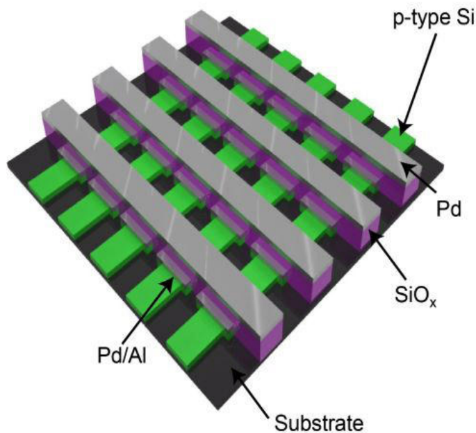
Рис.2 Комутаційна матриця
