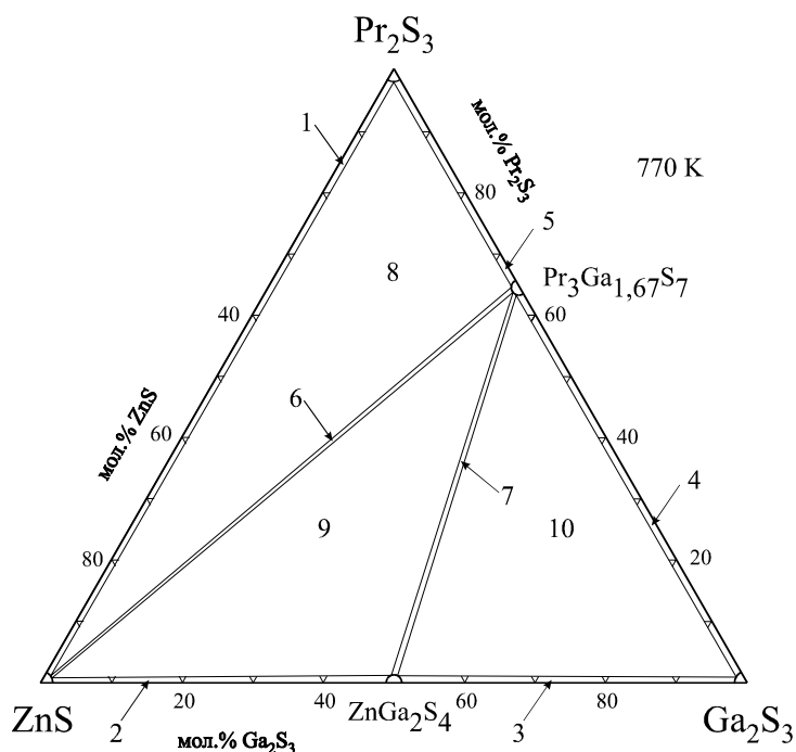
Рис. 1. Ізотермічний переріз системи \text{ZnS} - \text{Pr}_2\text{S}_3 - \text{Ga}_2\text{S}_3 за температури 770 K: 1 – \text{ZnS} + \text{Pr}_2\text{S}_3 ; 2 – \text{ZnS} + \text{ZnGa}_2\text{S}_4 ; 3 – \text{Ga}_2\text{S}_3 + \text{ZnGa}_2\text{S}_4 ; 4 – \text{Ga}_2\text{S}_3 + \text{Pr}_3\text{Ga}_{1,67}\text{S}_7 ; 5 – \text{Pr}_2\text{S}_3 + \text{Pr}_3\text{Ga}_{1,67}\text{S}_7 ; 6 – \text{ZnS} + \text{Pr}_3\text{Ga}_{1,67}\text{S}_7 ; 7 – \text{ZnGa}_2\text{S}_4 + \text{Pr}_3\text{Ga}_{1,67}\text{S}_7 ; 8 – \text{Pr}_2\text{S}_3 + \text{ZnS} + \text{Pr}_3\text{Ga}_{1,67}\text{S}_7 ; 9 – \text{ZnS} + \text{ZnGa}_2\text{S}_4 + \text{Pr}_3\text{Ga}_{1,67}\text{S}_7 ; 10 – \text{Ga}_2\text{S}_3 + \text{ZnGa}_2\text{S}_4 + \text{Pr}_3\text{Ga}_{1,67}\text{S}_7 .
