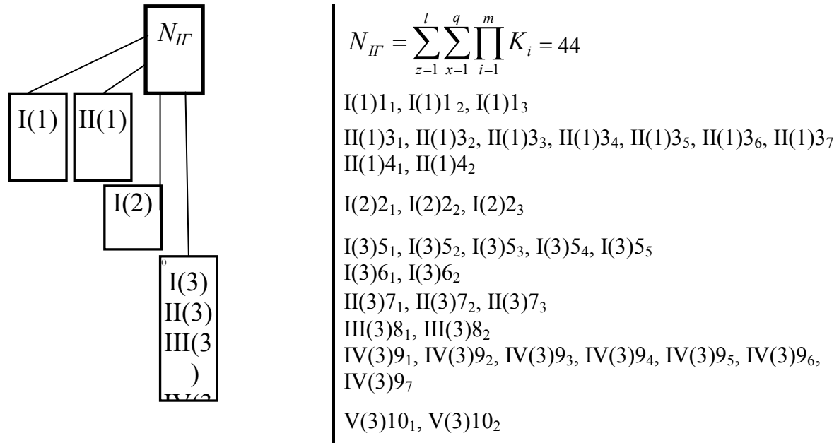
Рис. 1. Модель механічної системи «Конструктивних ознак та елементів процесу навивання гвинтових заготовок»: I – V – відповідні підгрупи ієрархічного рівня; (1)–(3) – відповідний ієрархічний рівень
