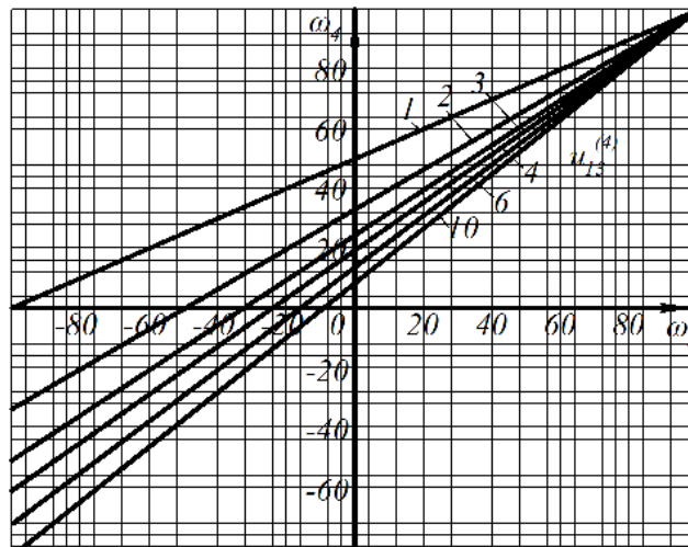
Рис. 2. Залежності \omega_4 = f(\omega_3, \omega_1, u_{13}^{(4)}) , при u_{13}^{(4)} = 1 \dots 10 і \omega_1 = 100 \text{ рад/с}
