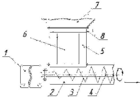
Рис. 1. Пристрій для дослідження процесу захоплення сипучих вантажів конічними шнеками
