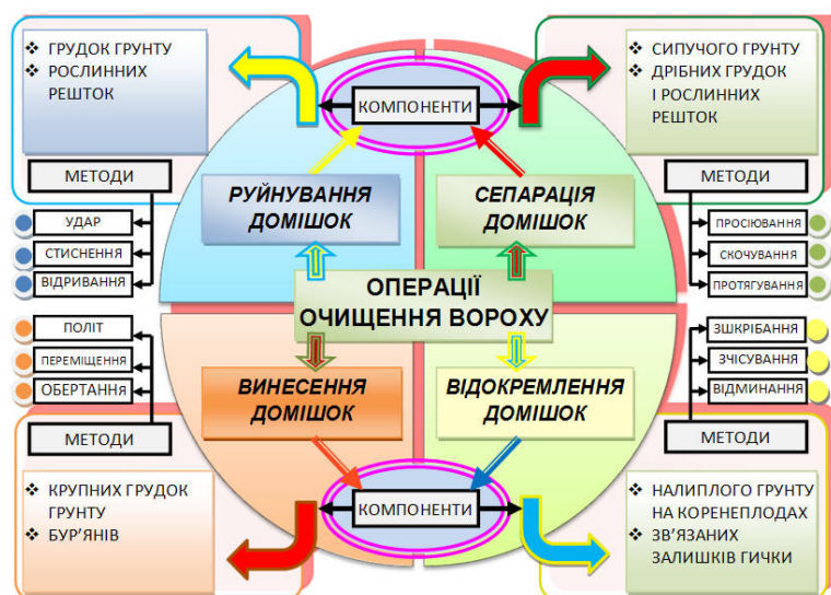
Рис. 3. Операції очищення вороху
