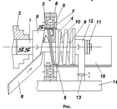
Рис. 2. Спосіб навивання спіралі щільним пакетом
