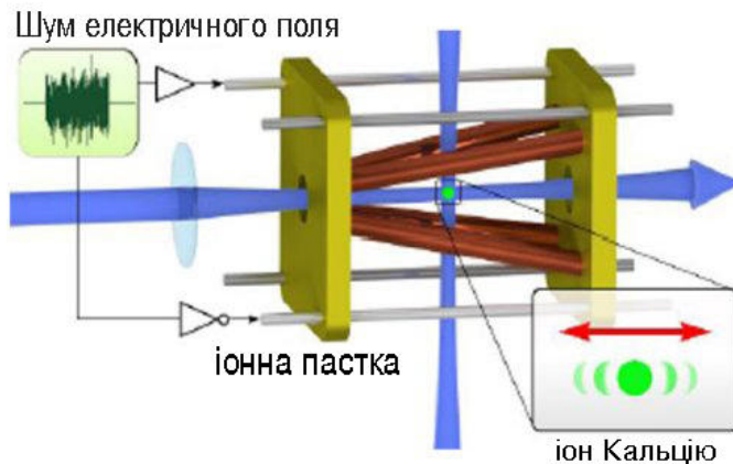
Рис 1. Принцип роботи атомарного теплового двигуна.
