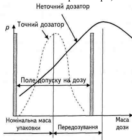
Рис. 1. Вплив точності дозатора на витрати продукту
