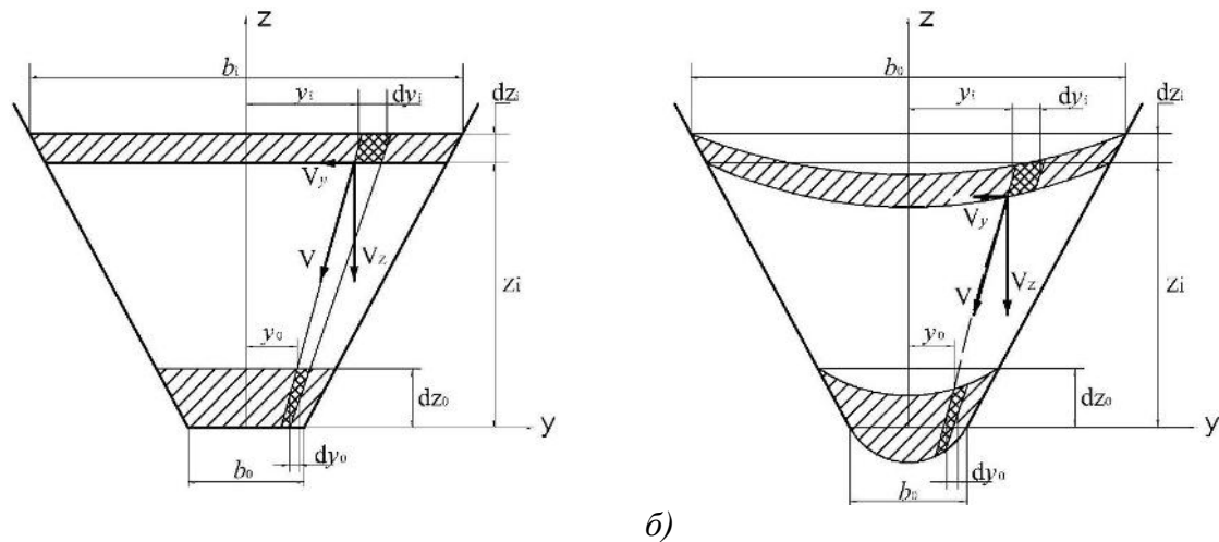
Рис. 1. Схема до визначення деформації витoku вантажу з паралельним зсувом шарів матеріалу (а) та із врахуванням тертя матеріалу до стінок жолоба (б). У першому випадку прийнято, що деформація проходить рівномірно, тобто для кожного елементарного об'єму з однаковою координатою z буде однакова деформація. Якщо матеріал при русі у просторі бункера не ущільнюється і не розріджується то, для довільного виділеного елементарного об'єму A_i з координатами y_i та z_i , умова нерозривності сипкого матеріалу має вигляд: \dot{\varepsilon}_y + \dot{\varepsilon}_z = 0 , де \varepsilon_y, \varepsilon_z - деформації виділеного об'єму вантажу за відповідними координатами, \varepsilon_y = dy/y , \varepsilon_z = dz/z .
