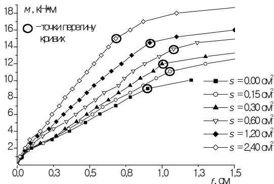
Рис. 3. Прогини зразків з різною площею перерізу ( S ) підсилювальної стрічки за квазістатичного навантаження
