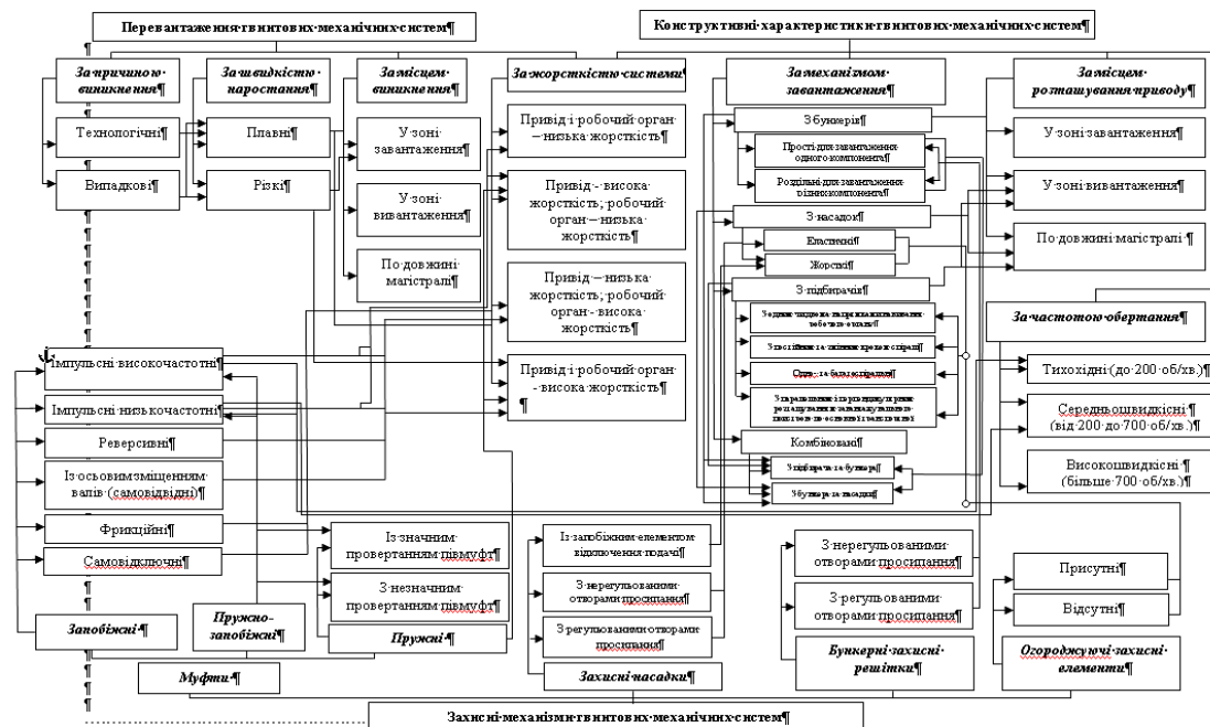
Рисунок 1 - Взаємозв'язок елементів гвинтових механізмів з характером навантаження
