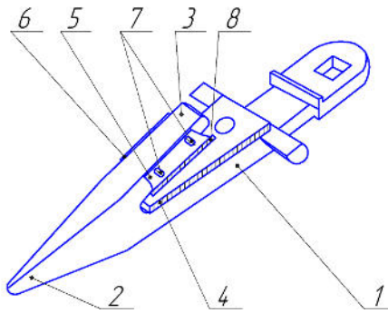
Рис. 1. Палець різального апарату
