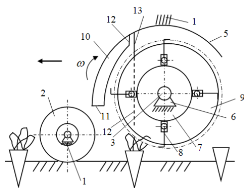
Рис. 2. Конструктивна схема гичкозбирального модуля
