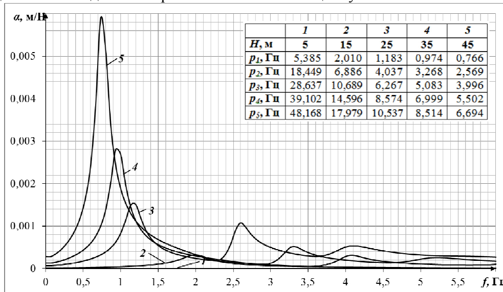
Рис. 1. Локальні динамічні податливості тягового органу ескалатора: p_i - власні частоти, Гц; H - висота підйому, м
