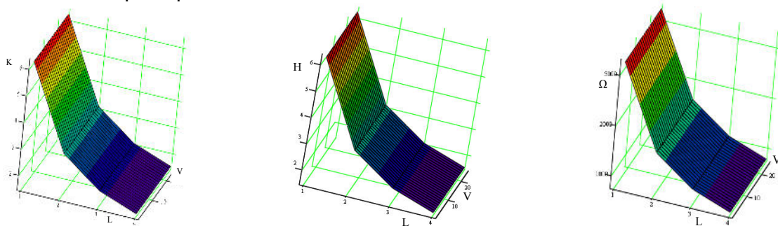
Рис.1. Залежність хвильових чисел та частоти від швидкості руху робочого органу та довжини
