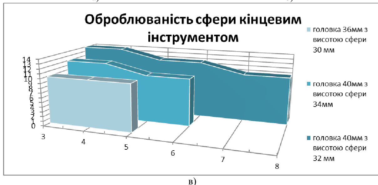
Ри.1. Моделювання оброблення: а) початок оброблення, б) завершення оброблення (варіант з позитивним результатом), в) діаграма співвідношення діаметру інструменту та товщини стінки оболонки, при яких схема контакту «інструмент-поверхня» нерозривна
