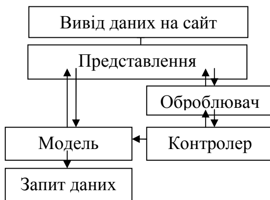
Рисунок 1 – Узагальнена структурна схема MVC Zend Framework
