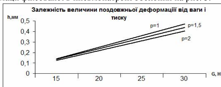
Рис. 2 . Залежність деформації оболонки від ваги пляшки для різного тиску в пневмосистемі
