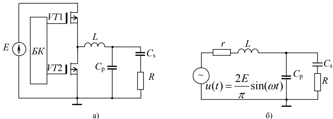
Рисунок 1 - Резонансний інвертора (а) та його еквівалентна схема (б)
