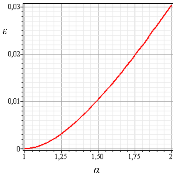
Рисунок 3 - Залежність максимального відносного відхилення потужності від діапазону зміни навантаження Figure 3 – maximum relative power deviation vs. load variation range
