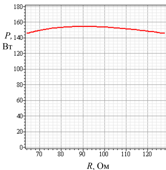
Рисунок 4 - Залежність потужності інвертора від опору навантаження Figure 4 – Inverter power vs. load resistance
