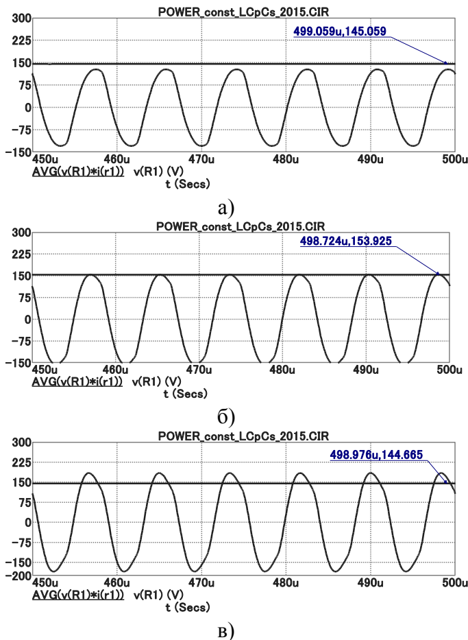
Рисунок 5 - Результати моделювання: а) для мінімального опору; б) для максимальної потужності; в) для максимального опору Figure 5 – Modeling results: a) for minimum resistance; б) for maximum power; в) for maximum resistance
