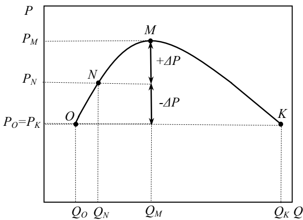
Рисунок 2 - Залежність відносної потужності резонансного інвертора від добротності Figure 2 – Resonant inverter relative power vs. quality factor
