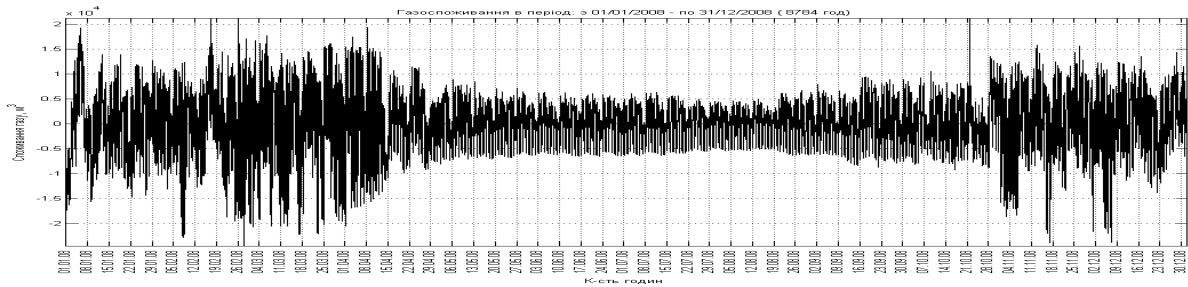
Рис.2 – Залишок після виділення тренду
