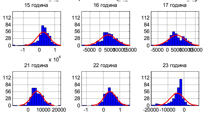
Рис.3 – Гістограмний аналіз фі-серій для залишку
