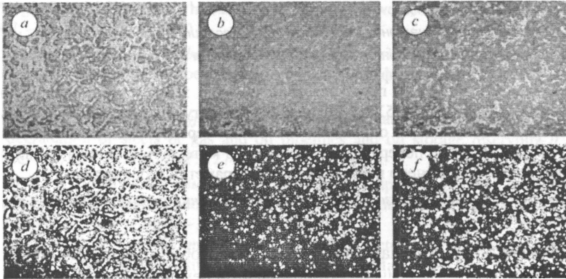
Рис. 1. Вихідні (a–c) та бінаризовані (d–f) зображення впорядкованих структур на поверхні сталі 15X13МФ після лазерного імпульсного оброблення на повітрі (a, d), у воді (b, e) і чорнилі (c, f).
