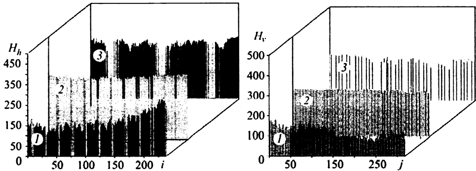
Рис. 2. Горизонтальна H_h (a) і вертикальна H_v (b) гістограми інтегральних інтенсивностей бінарних зображень впорядкованого рельєфу поверхонь зразків сталі 15X13MF після їх лазерного імпульсного оброблення на повітрі (1), у воді (2) і чорнилі (3).
