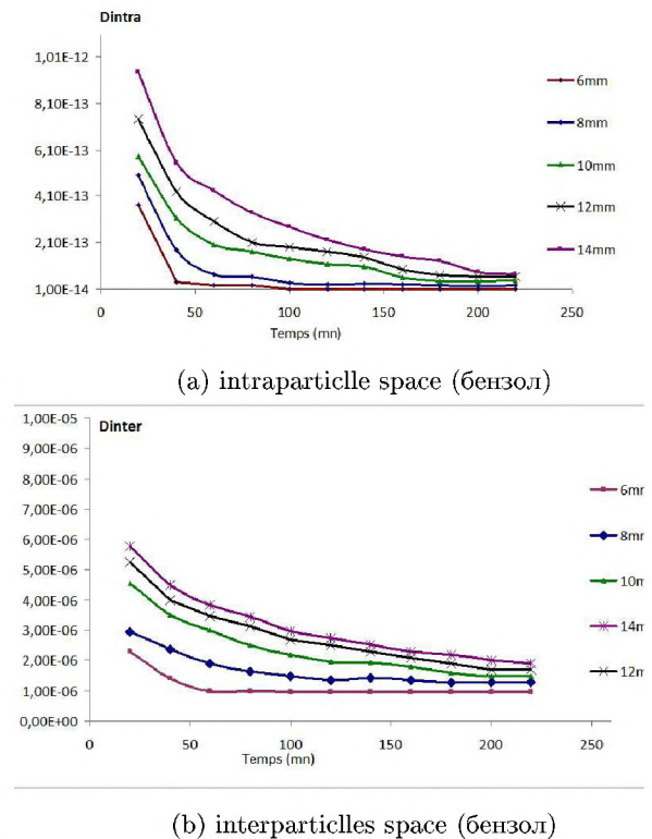
Рис. 1: Профілі коефіцієнтів дифузії бензолу
