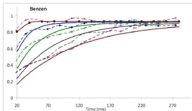
(a) бензол
