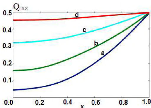
(b) гексан(8мм)
