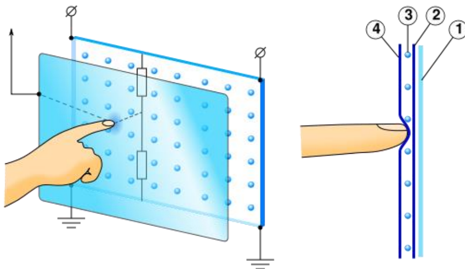
Рисунок 10.7 – Принцип дії резистивного сенсорного екрану
