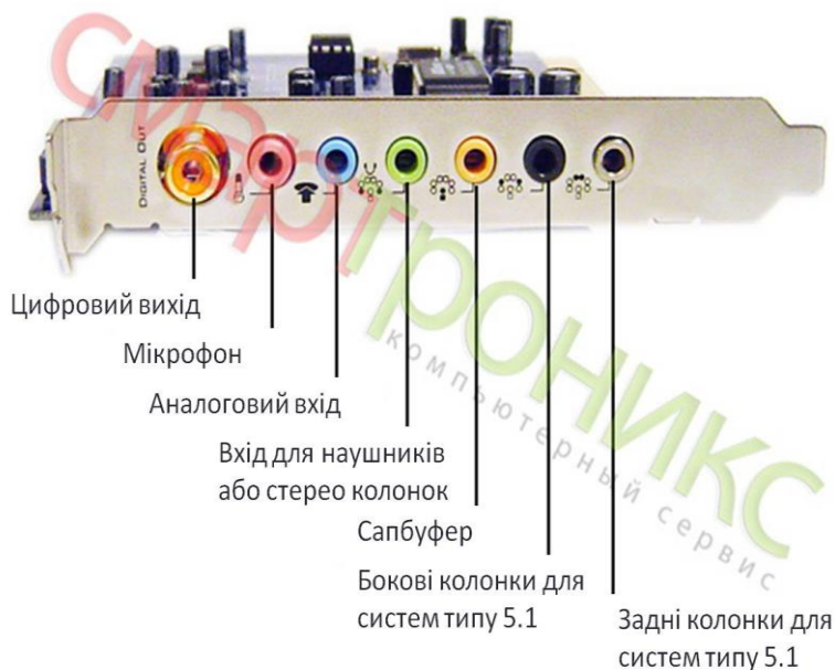
Рисунок 8.3 - Типи роз'ємів звукової карти
