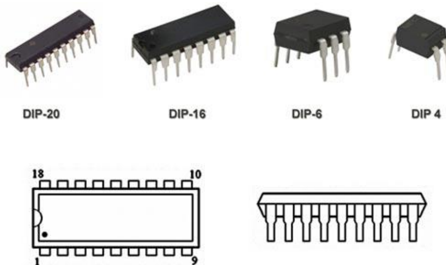
Рисунок 7.1 - Модулі пам'яті DIP
