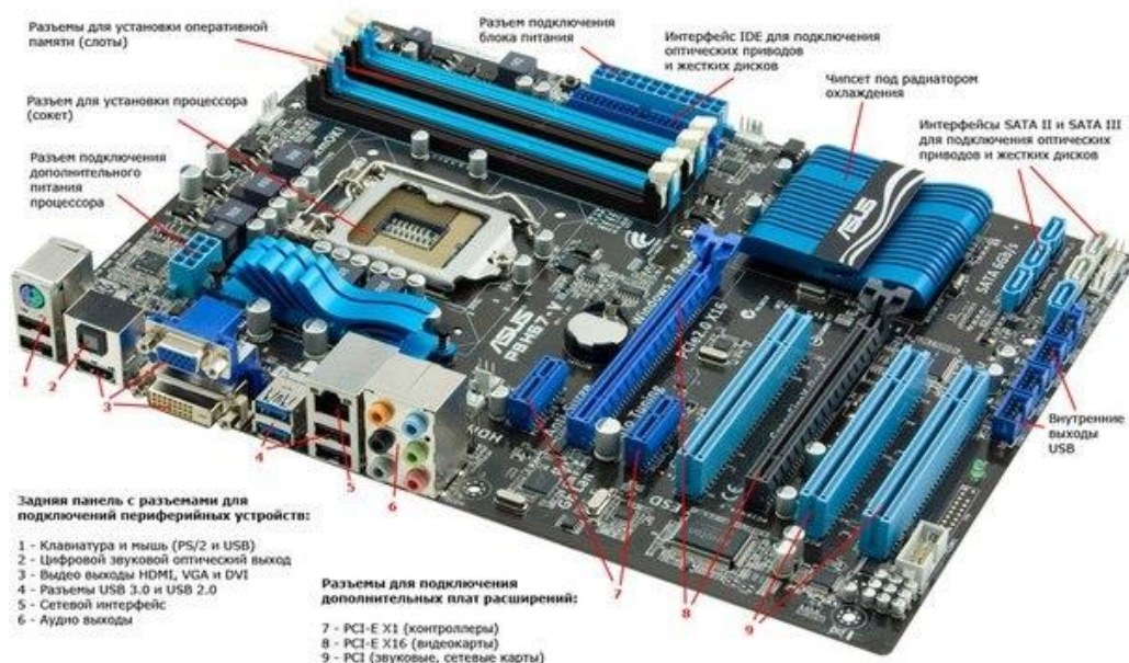
Рисунок 5.1 - Зовнішній вигляд материнської плати
