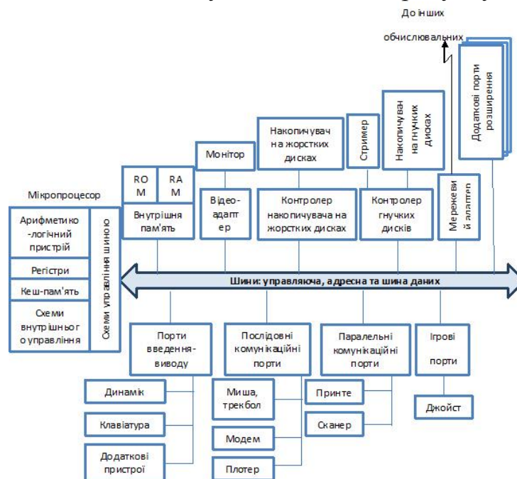
Рисунок 3.3 – Загальна структура персонального комп'ютера
