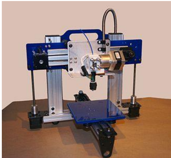
Рисунок 10.20 – 3D-принтер
