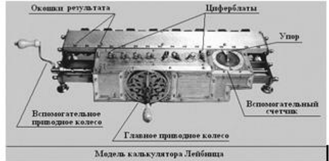
Рисунок 1.3 – Модель ступінчастого обчислювача Лейбніца
