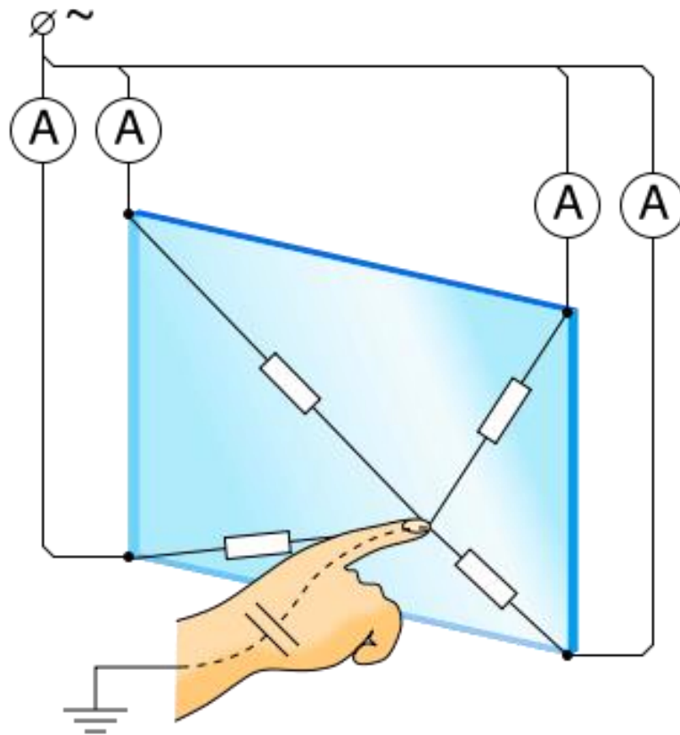
Рисунок 10.8 – Принцип дії ємнісного сенсорного екрану
