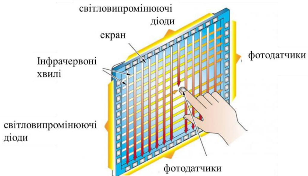
Рисунок 10.10 – Принцип дії інфрачервоного екрану
