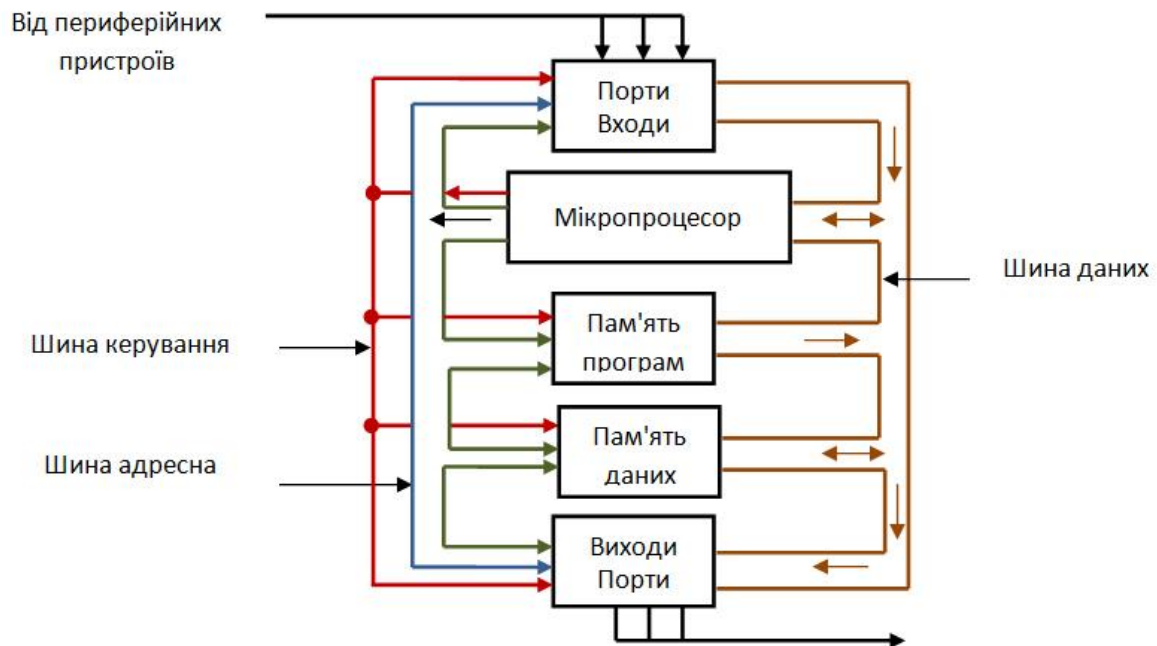
Рисунок 6.2 – Архітектура типового мікропроцесору
