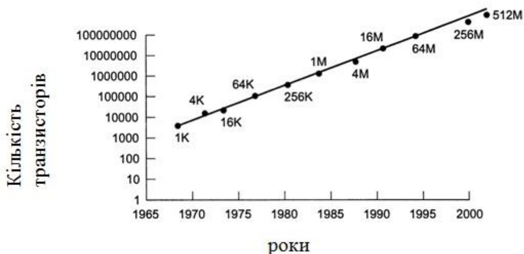
Рисунок 2.1 – Графічне відображення закону Мура
