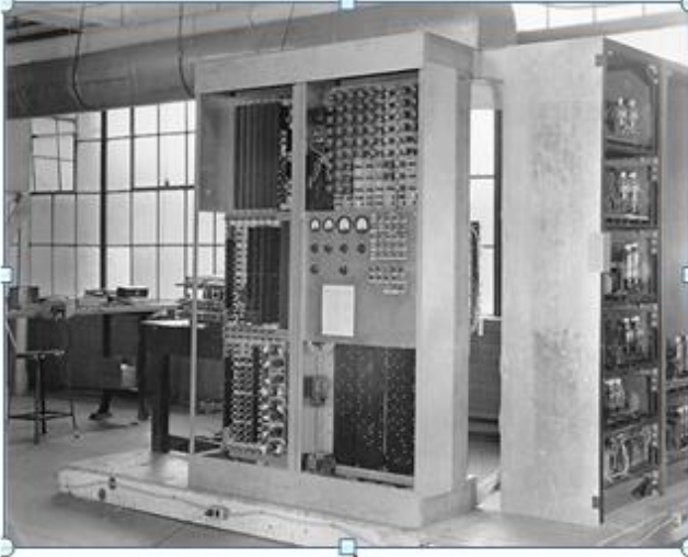
Рисунок 1.8 – Представники I-го покоління ЕОМ: а) Electronic Discrete Variable Computer ; б) Universal Automatic Computer
