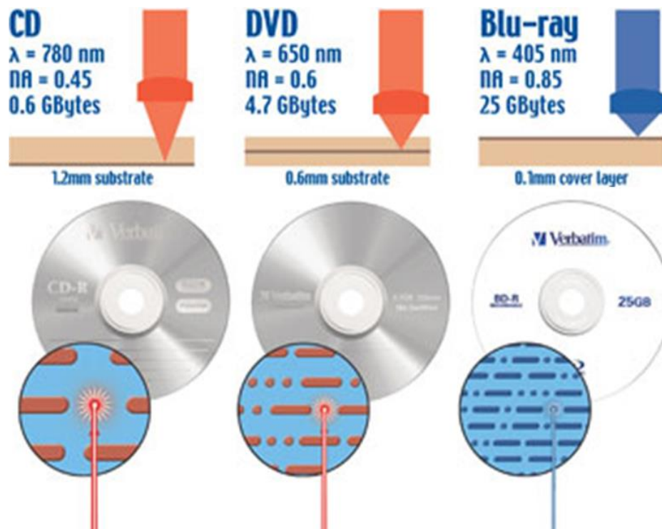
Рисунок 11.3 — Ілюстрація відмінностей в технологіях оптичних носіїв
