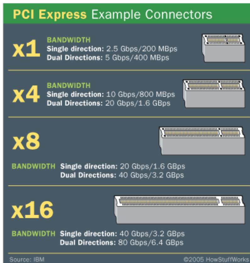
Рис. 8.2. Приклад слотів з різною кількістю ліній
