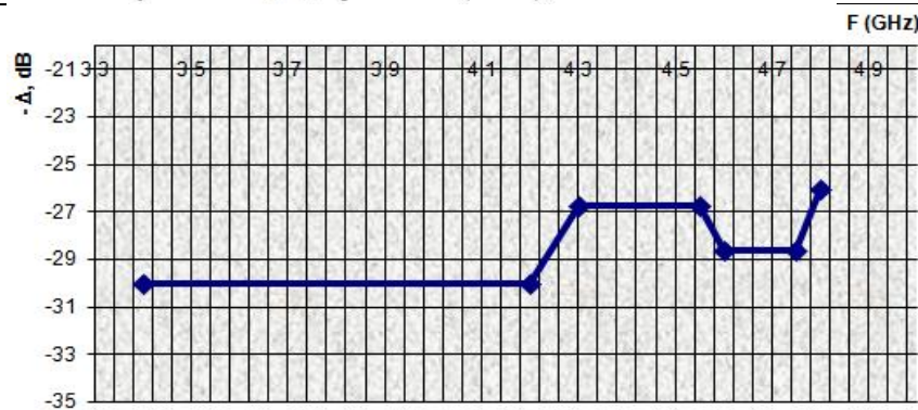
Рисунок 5- Обвідна діаграма поляризаційної розв'язки Е/Н
