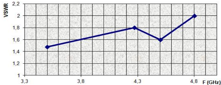
Рисунок 4 - Обвідна діаграма КСХн (VSWR), боковий канал
