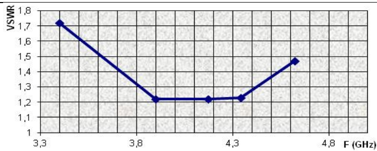
Рисунок 3 - Обвідна діаграма КСХн (VSWR), прямий канал Н
