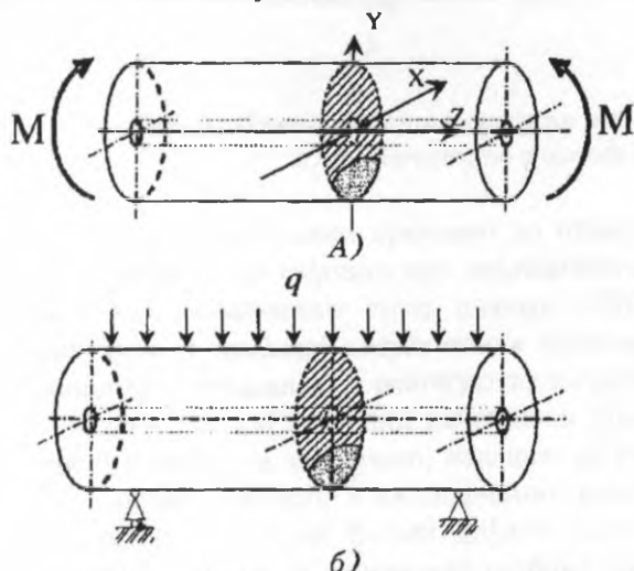
Рис. 1. Схеми навантажування товстостінного циліндра з тріщиною: а) – чистий згин; б) – рівномірно розподілене навантаження
