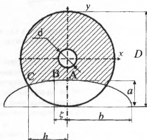
Рис. 2. Геометрія тріщини
