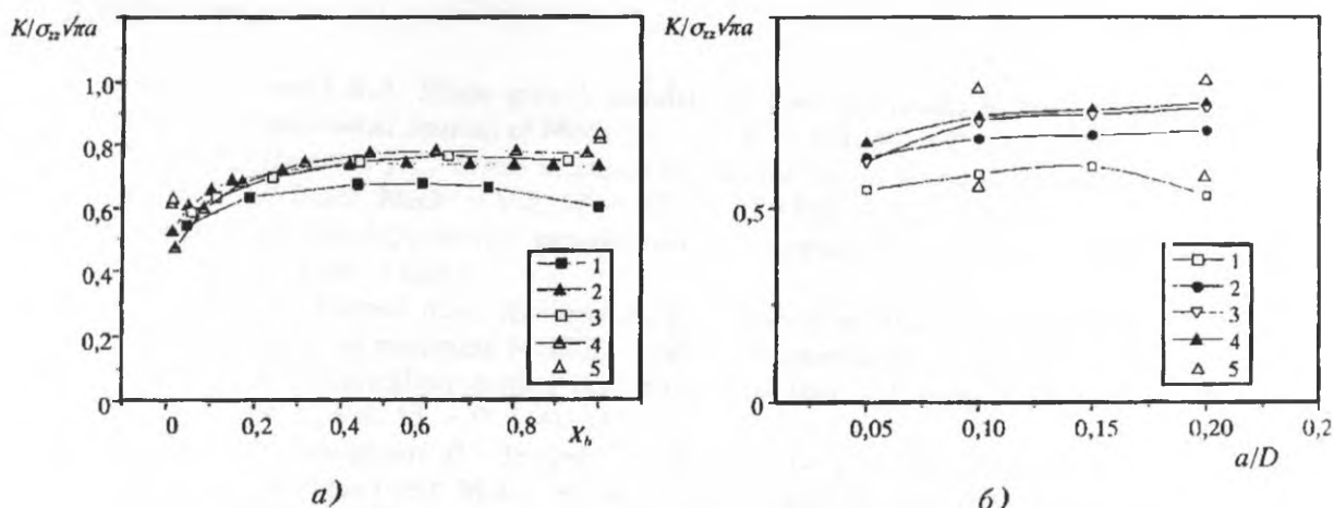
Рис. 6. Залежність нормалізованих КІІ товстостінного циліндра з поверхневою напівеліптичною тріщиною від параметра X_b - a ,
