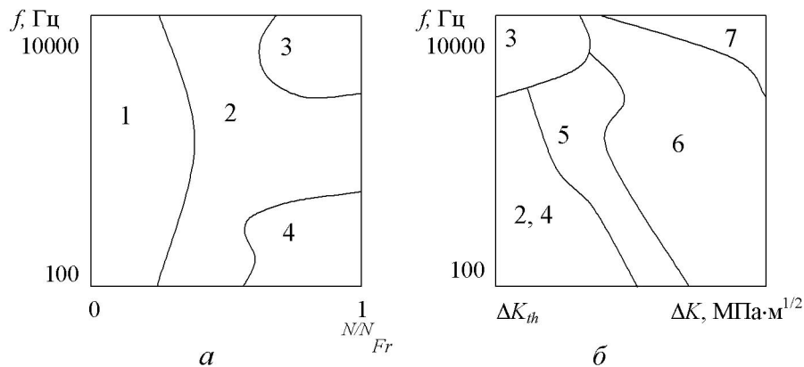
Рис. 1. Схематическое представление преобладающих типов дислокационных структур в титановых сплавах на стадии накопления усталостных повреждений ( a ) и на стадии стабильного роста трещины ( б ): 1 – границы наклона, сетки, одиночные дислокации; 2 – деформация межфазных границ; 3 – дефекты упаковки; 4 – петли; 5 – плоские скопления, ячеистая структура; 6 – полосовая структура; 7 – деформация микрообластей, прилегающих к исходно присутствующим в \alpha - фазе двойникам.
