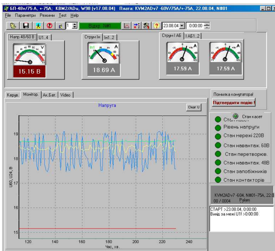
Рисунок 3 – Інтерфейс програми моніторингу джерела гарантованого живлення
