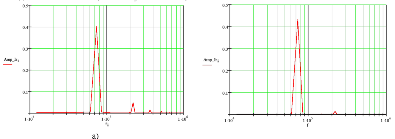
Рис.2. Спектральні характеристики вихідного струму ПТ при навантаженні ЛЛ (а) та активним опором R_n=150 \text{ Ом} (б).
