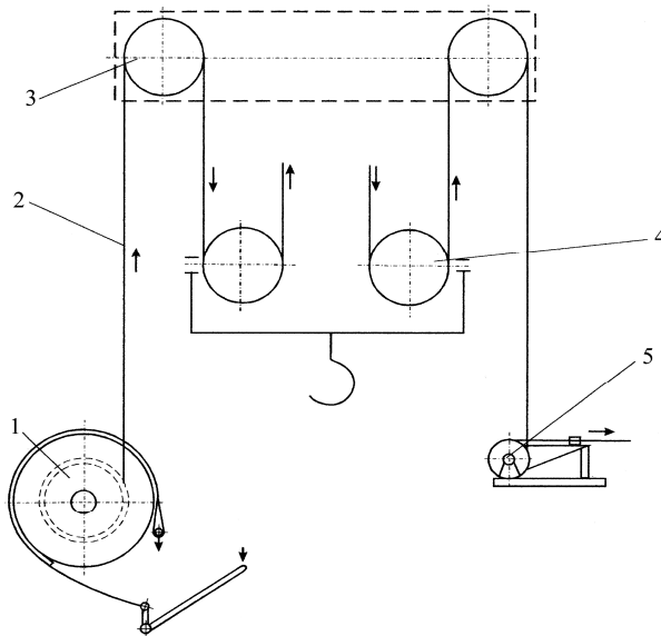
Схема обмеженого зворотного перепуску талевого каната в талевій системі бурової установки:
