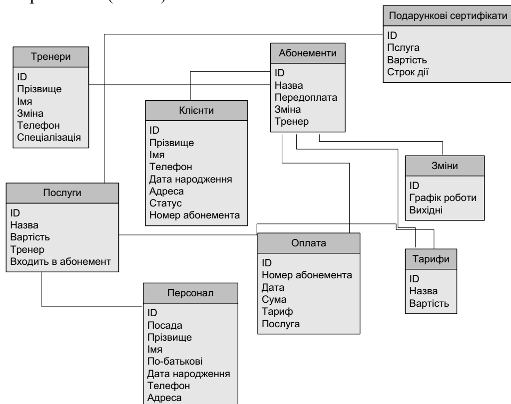
Рис. 1. Модель бази даних
