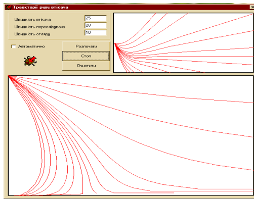
Рис. 2 До аналізу залежностей відстаней між втікачем та переслідувачем від часу
