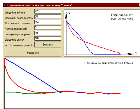
Рис.1 Комп'ютерне моделювання С-стратегії (криві) та Л-стратегії (прямі лінії)
