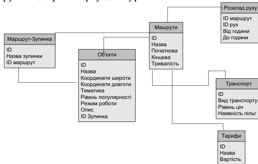
Рис. 1. Модель бази даних
