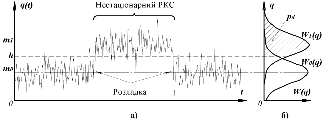
Рис. 7 Залежність імовірності правильного визначення розладки РКС p_d від порогу визначення h : а) тестова статистика визначення q , б) густина розподілу W(q) імовірності тестової статистики q .
