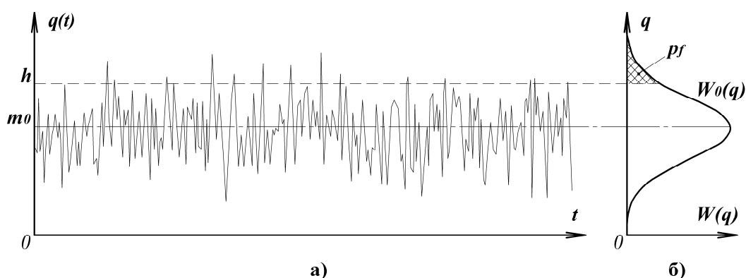
Рис. 6 Залежність імовірності помилкового визначення розладки РКС p_f від порогу визначення h : а) тестова статистика визначення q , б) густина розподілу W(q) імовірності тестової статистики q .
