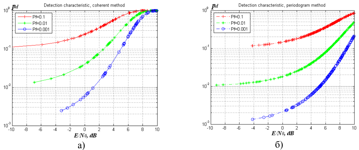
Рис. 13. Характеристики достовірності визначення розладки РКС, обчислені за спектральними компонентами отриманими: а) синфазним методом, б) методом періодограм,
