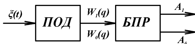
Рис.5 Структурна схема визначення розладки РКС: \xi(t) — спостережуваний РКС, W_0(q) , W_1(q) — густина розподілу імовірності тестової статистики q стаціонарного та ПКВП РКС при розладці на виході ПОД, БПР— блок прийняття рішення, A_0 або A_1 — прийняте рішення про стаціонарність або про розладку РКС.
