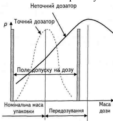
Рис. 1. Вплив точності дозатора на витрати продукту
