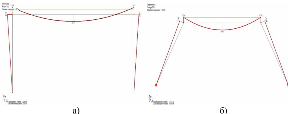
Рис.1. Згинальні моменти в рамах з одиничним навантаженням:
