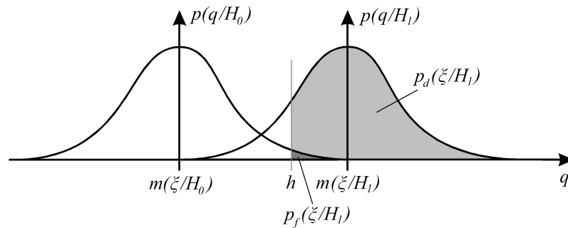
Рис. 1. Густини розподілу ймовірностей p(q/H_1) і p(q/H_0) ЕКС
